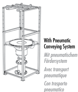
With Rotary Valve Mit Zellenradschleuse Avec sas alvéolaire Con rotavalvola
